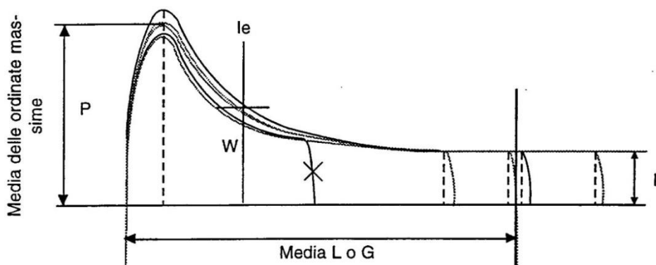
Figura 1 Curva tipica di un alveogramma
